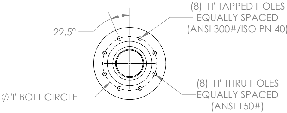
4" DISCHARGE FLANGE DETAIL ANSI 150# ANSI 300# ISO/DIN PN40
