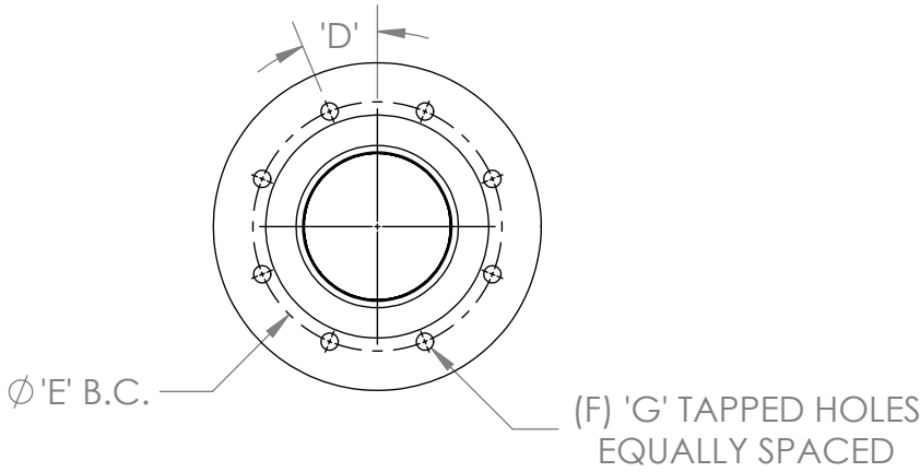
6" SUCTION FLANGE DETAIL ANSI 150# ANSI 300# ISO/DIN PN40
