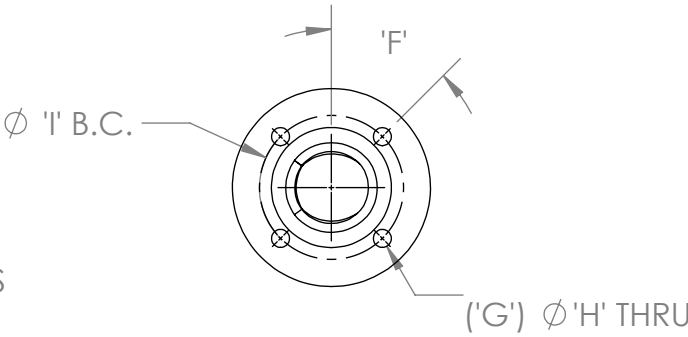
3" DISCHARGE FLANGE DETAIL ANSI 150# ANSI 300# ISO/DIN PN40
