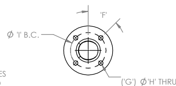
3" DISCHARGE FLANGE DETAIL ANSI 150# ANSI 300# ISO/DIN PN40
