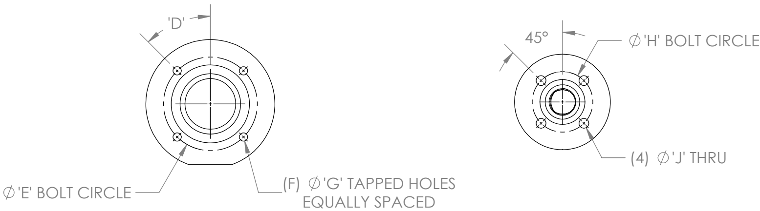
3" SUCTION FLANGE DETAIL ANSI 150# ANSI 300# ISO/DIN PN40
