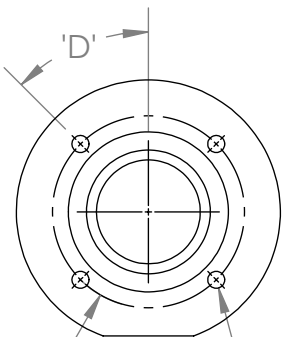
3" SUCTION FLANGE DETAIL ANSI 150# ANSI 300# ISO/DIN PN40
