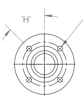
2" DISCHARGE FLANGE DETAIL ANSI 150# ANSI 300# ISO/DIN PN40
